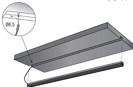
6010001 Clip di fissaggio (incluso) Fixing clip (included) Befestigungsclip (inbegriffen)
