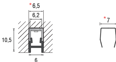
6010001 Clip di fissaggio (incluso) Fixing clip (included) Befestigungsclip (inbegriffen)
